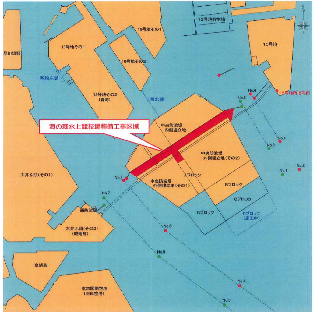
位置図（図-1）
